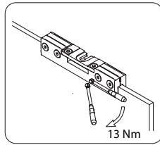
Fijación a vidrio
