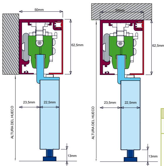
• COLOCACIÓN GUÍA A PARED
