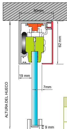
• COLOCACIÓN GUÍA A TECHO
