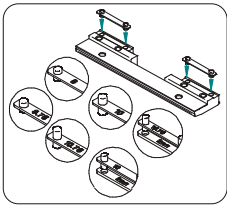
Separadores para vidrio de 8 a 12,76 mm
