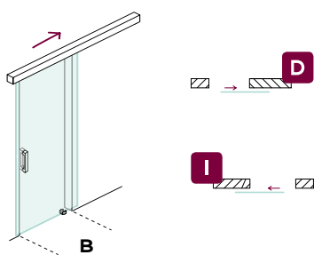
• COLOCACIÓN GUÍA A PARED
