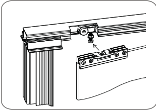
Montaje al perfil del cassonetto
