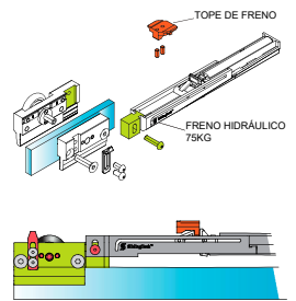
• PINZAS DE FIJACIÓN CON FRENO
