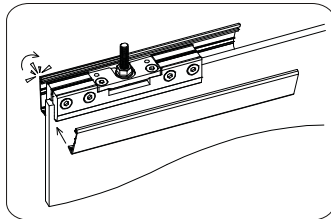
Montaje tapetas embellecedoras
