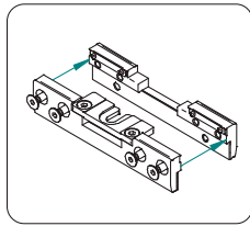
Montaje pinza
