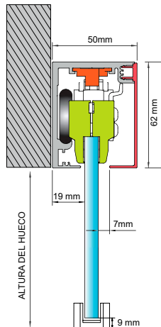
• COLOCACIÓN GUÍA A PARED
