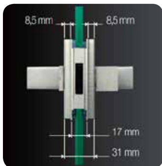
• MEDIDAS CERRADURA MAGNÉTICA
